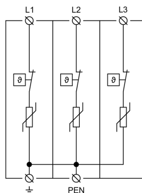
Vnútrotná schéma zapojenia
